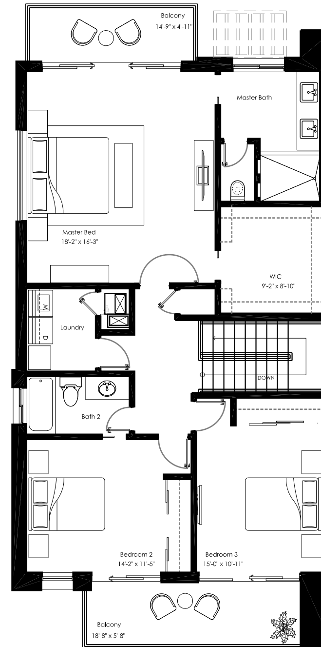
D1 SECOND FLOOR
