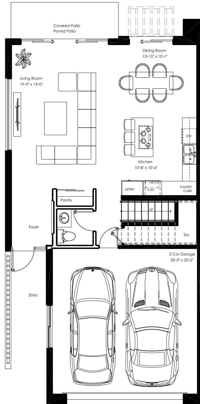
D1 FIRST FLOOR
